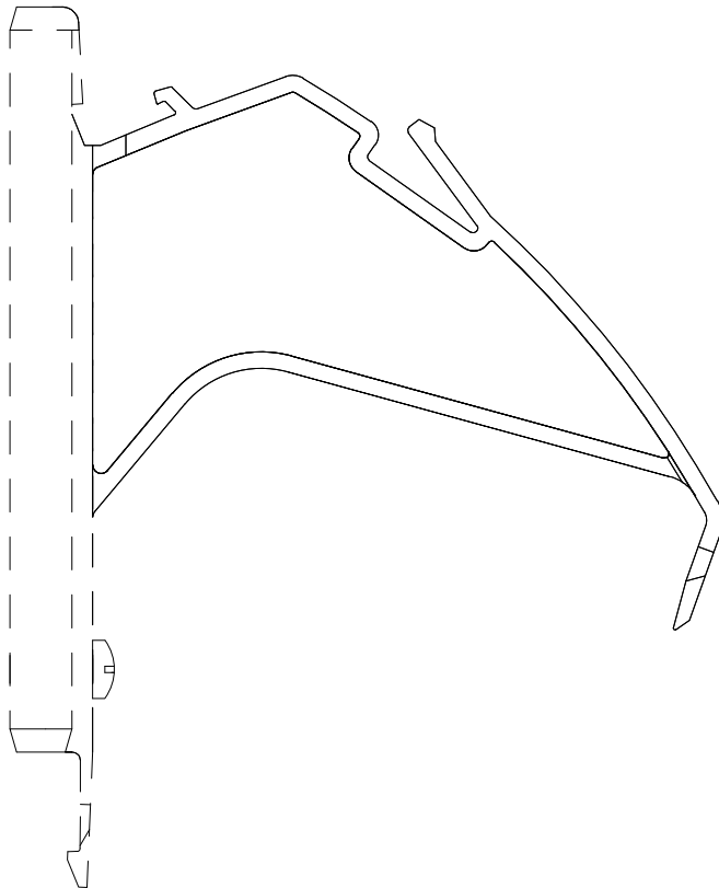
31 0904 0002 VERTICAL BRACKET 100R 45°
