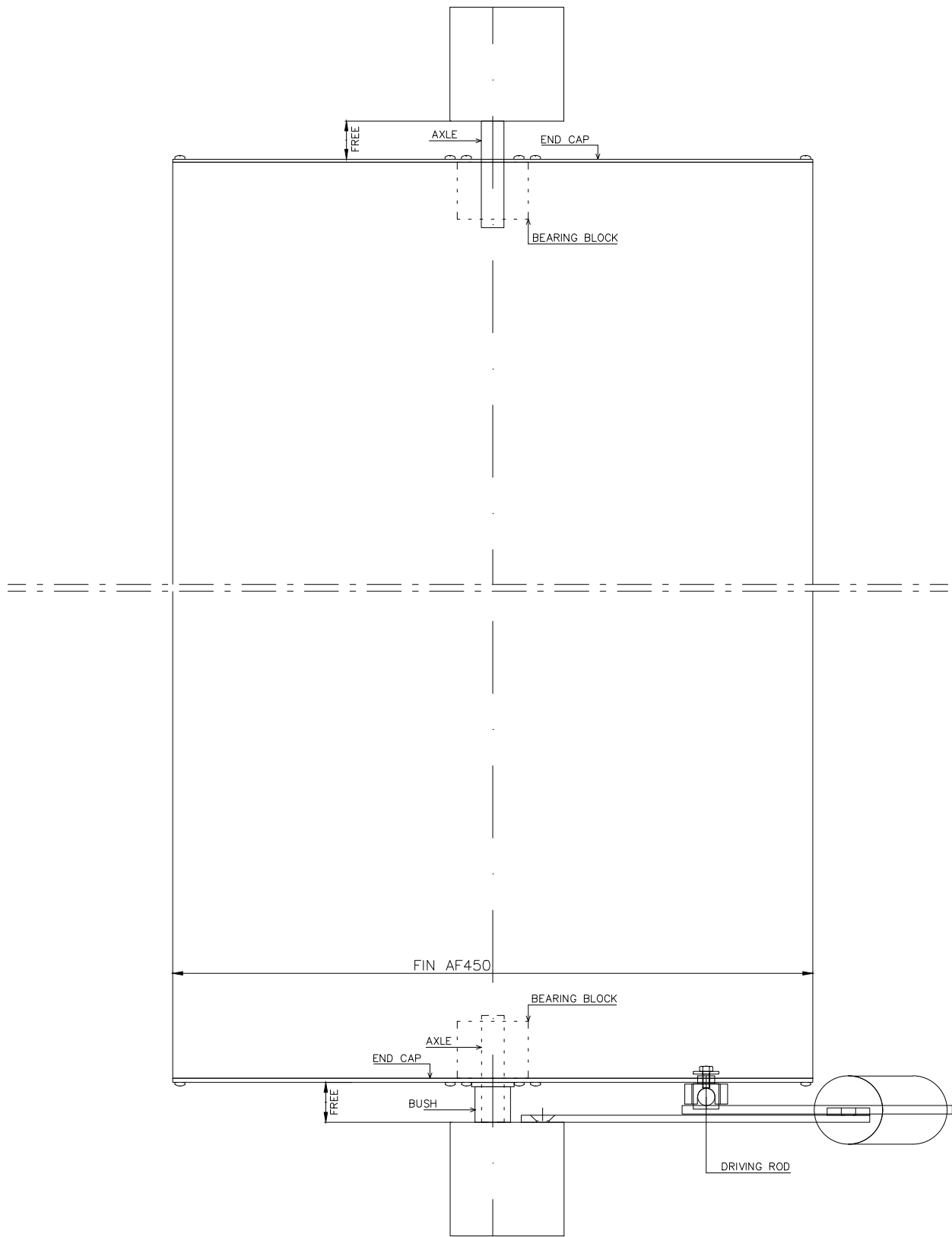
VERTICAL FIN450
