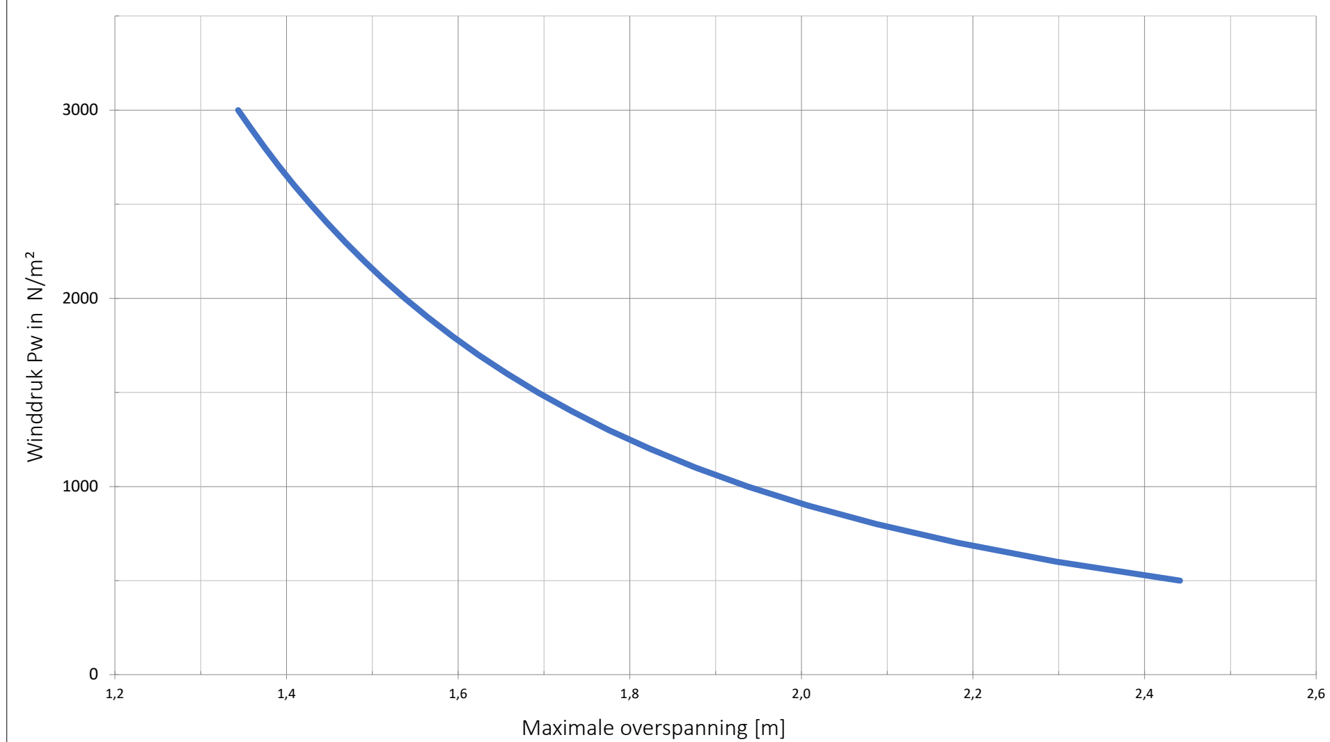
110-TC - Maximale afstand tussen 2 dragers
