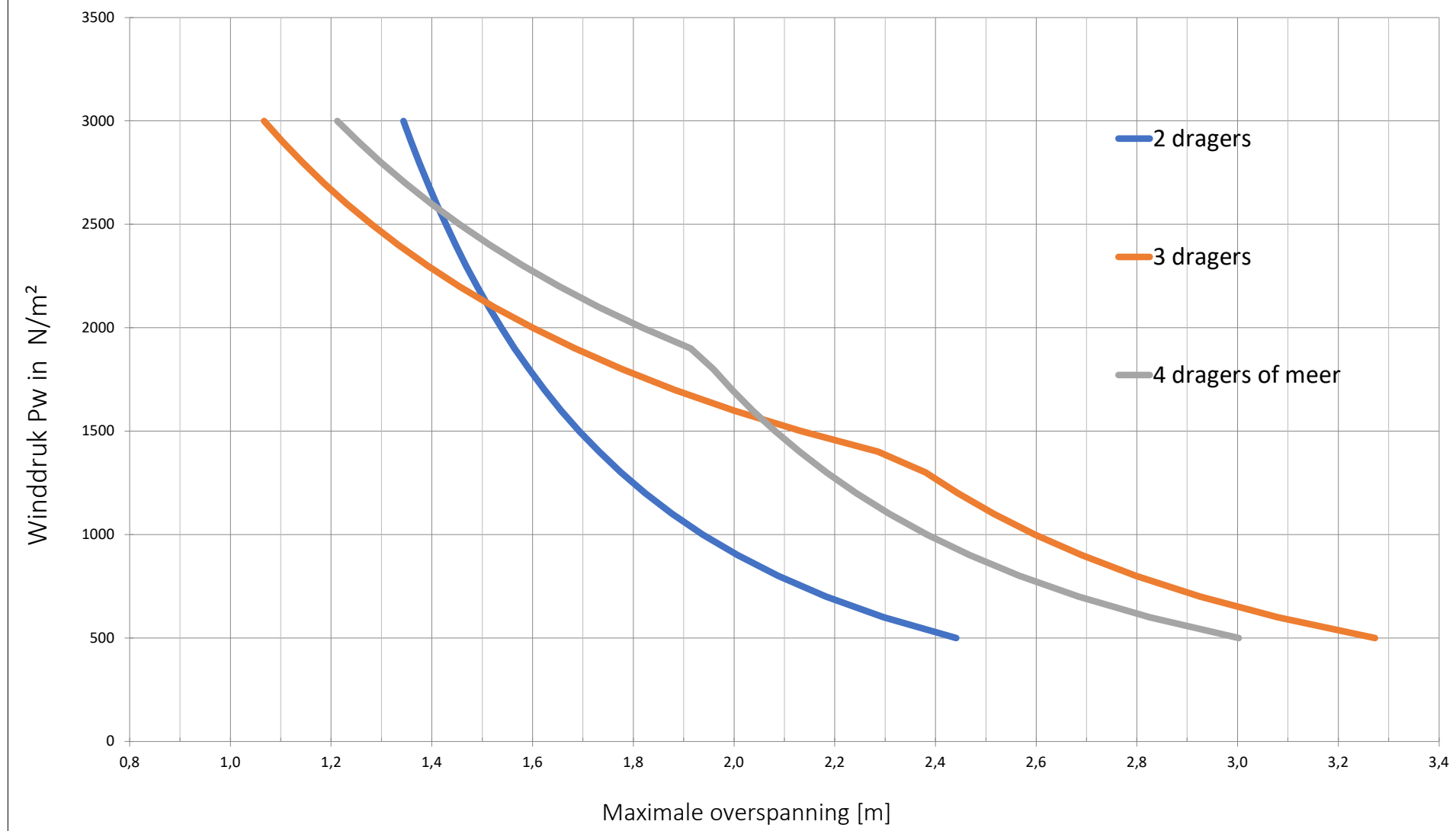
100-UC - Maximale afstand tussen de draagprofielen
